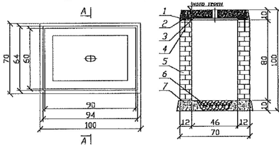
ДЕТАЙЛ - ШАХТА 60/90
